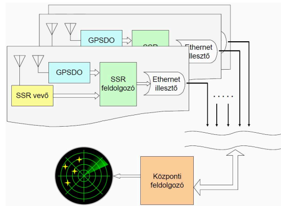
2. ábra Rendszer blokkvázlat
