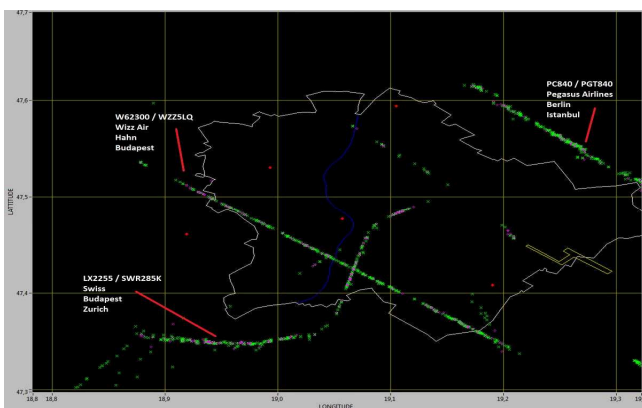
4. ábra Mode-S üzeneteken alapuló multilateráció
