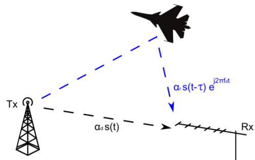
1. ábra Passzív radar jelútjai egyszerűsített modell szerint
