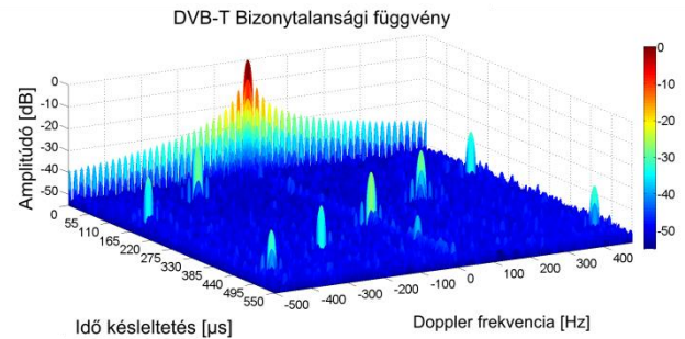
2. ábra A DVB-T jel bizonytalansági függvénye
