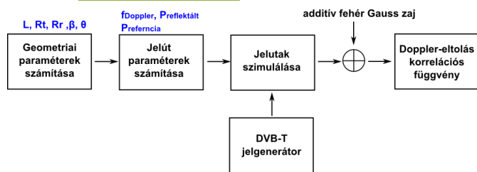
3. ábra Szimulációs program blokkdiagramja
